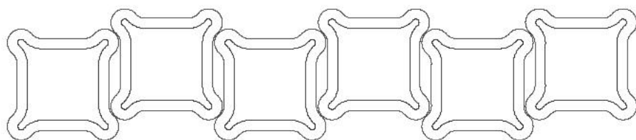
schema di posa 3 / laying scheme 3 28,19 pcs·sqm
