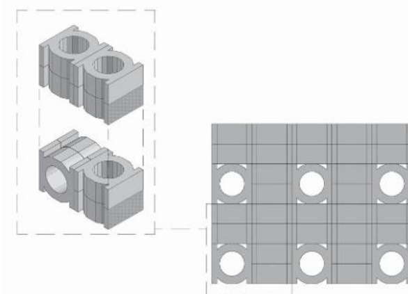
SCHEMA DI POSA 4 / LAYING SCHEME 4
