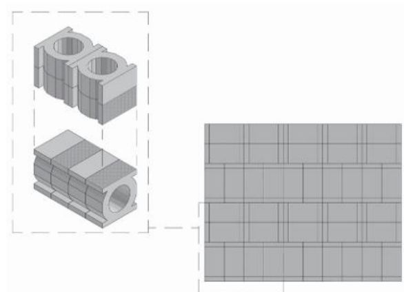
SCHEMA DI POSA 5 / LAYING SCHEME 5
