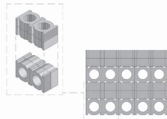
SCHEMA DI POSA 3 / LAYING SCHEME 3
