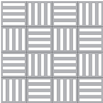
SCHEMA DI POSA 1 laying scheme 1
